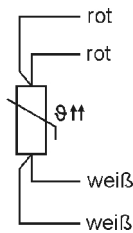
4-Leiter
