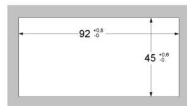
Schalttafel Ausschnitt gemäß DIN 43700-96x48
