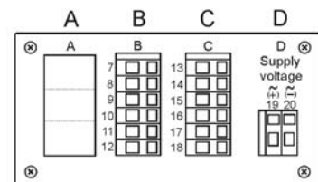
Anordnung der Anschlussleisten
